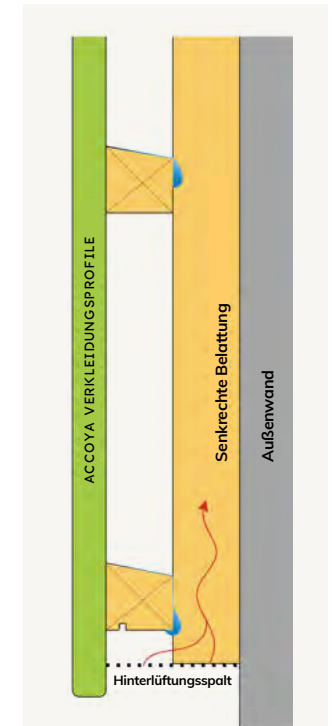
Abbildung 6: Doppelte Unterkonstruktion mit Ablaufrinne
