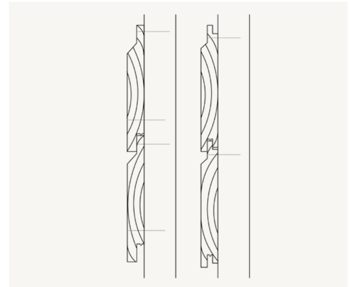
Abbildung 2: Abstandswulst
