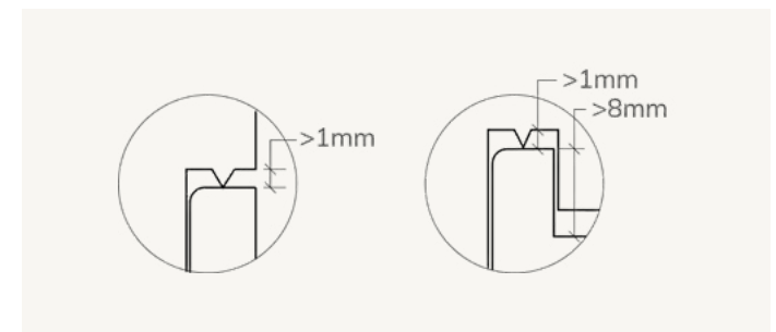
Abbildung 3: Abstandswulst (Detailansicht)
