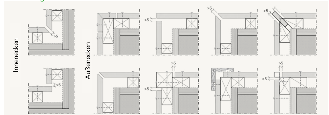
Abbildung 8: Ecklösungen; je nach örtlichen Bauvorschriften können Hohlraumabschottungen an den Ecken erforderlich sein.
